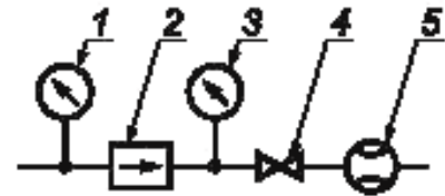
Рисунок 7 — Схема определения расходных характеристик предохранительных устройств
