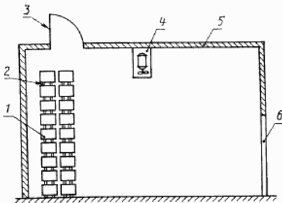
1—ящики; 2—деревянные бруски; 3—люк; 4—вентилятор; 5—потолок; 6—дверь
