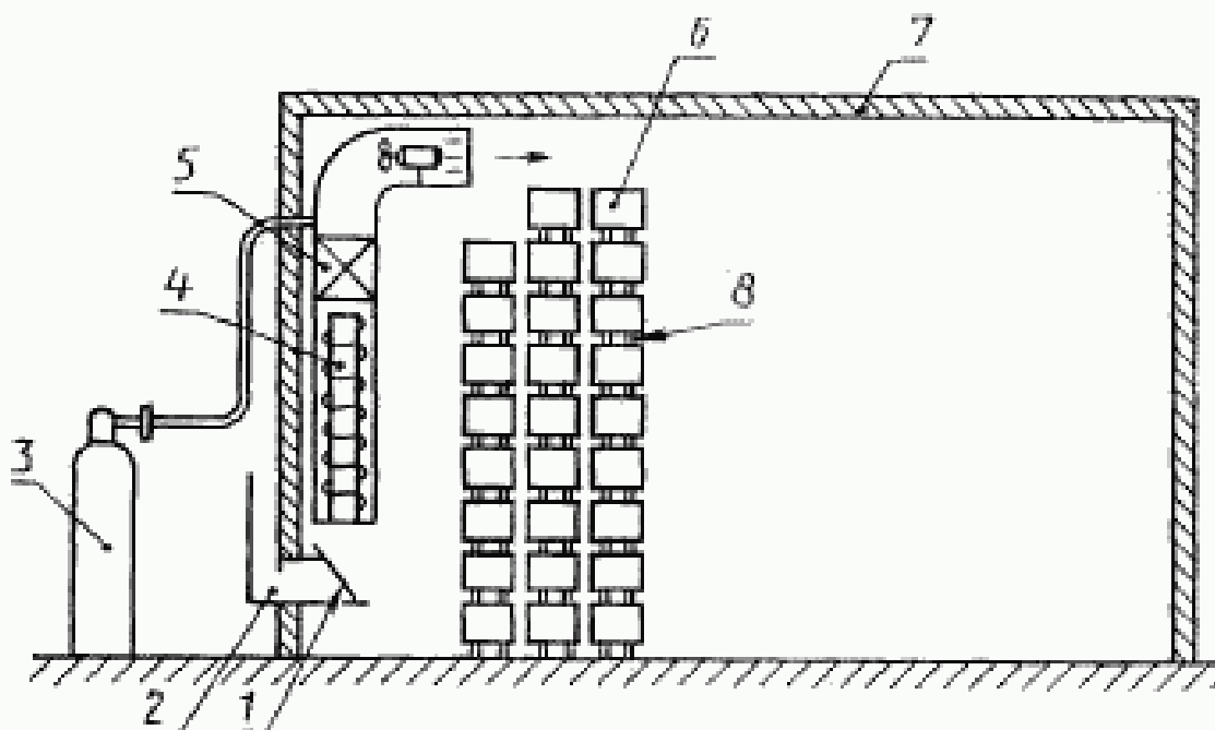
1—управляющий клапан; 2—выпускная труба; 3—газовый баллон; 4—охлаждающее устройство; 5—электрический нагреватель; 6—щитки; 7—потолок; 8—деревянные бруски
