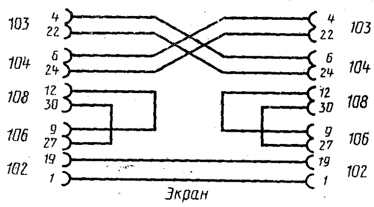
Соединение контактов
