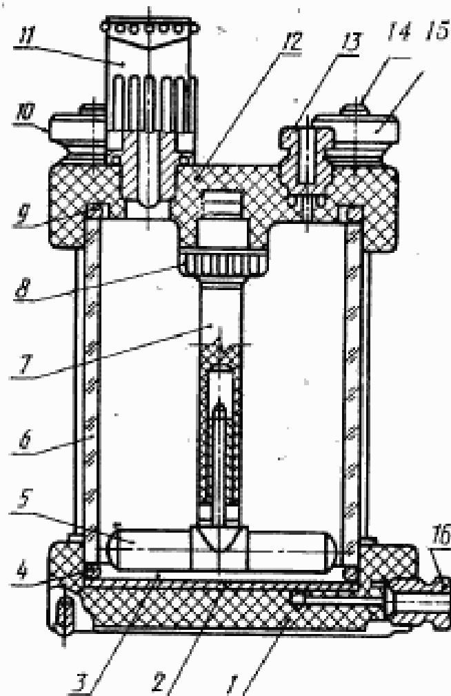
Схема ячейки для испытания мембран
