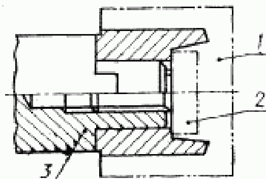
1—фреза; 2—стопорный ваят; 3—центрирующая часть оправки
