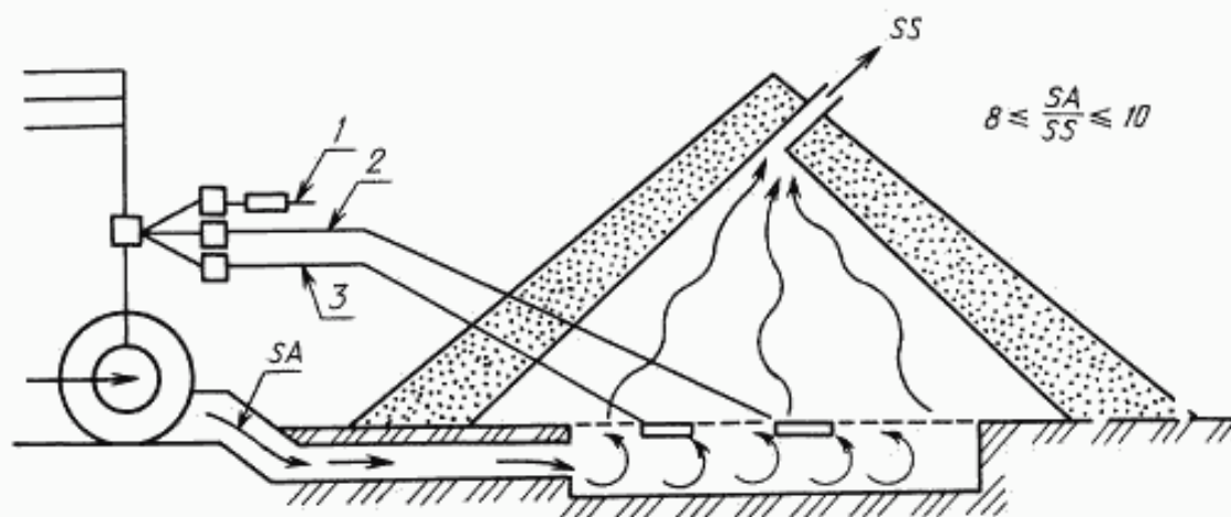
1, 2, 3 — регулирование тепловыми сигнальными устройствами; SA — поперечное сечение приточных труб; SS — поперечное сечение вытяжных труб
