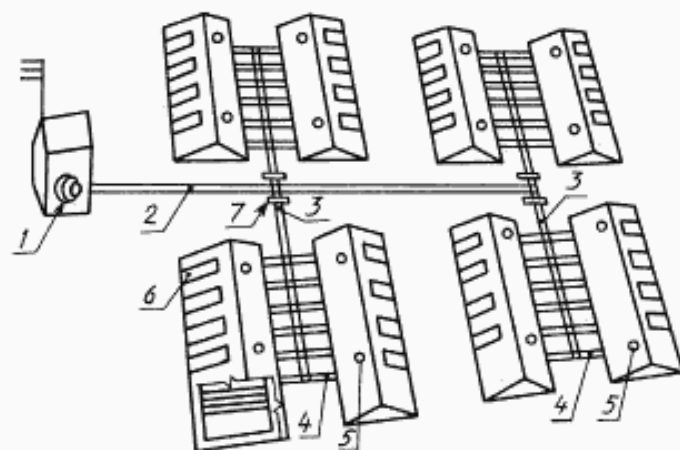
1 — вентилятор; 2 — центральный распределительный канал; 3 — боковые распределительные каналы; 4 — приточные трубы; 5 — вытяжные трубы; 6 — люк для загрузки; 7 — регулировочные заслонки
