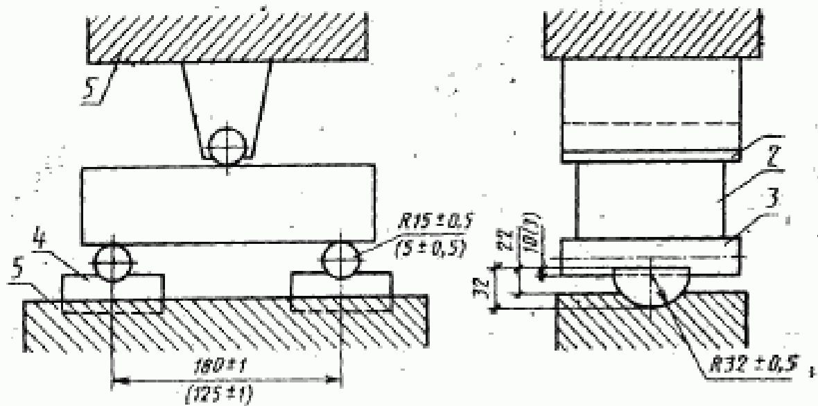
Схема нагружающего устройства
