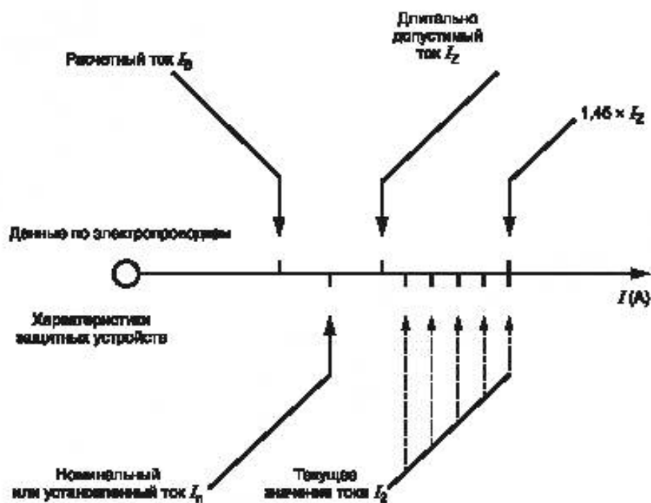
Рисунок В.1 — Иллюстрация условий 1 и 2 из 433.1
