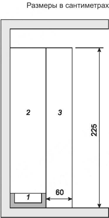
1 — зона 0; 2 — зона 1; 3 — зона 2
