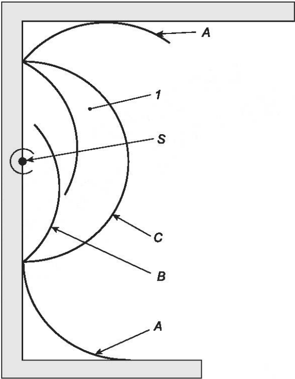
1 — зона 0 и зона 1; А — открытая душевая дверь; С — душевые двери при использовании душа; В — душевые двери, когда душ не используется; S — стационарный вентиль для воды
