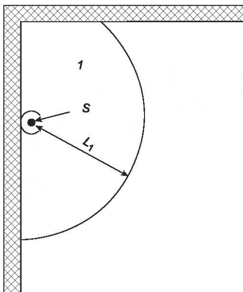
Рисунок 8 — Размеры зон 0 и 1: вид сверху на душ со стационарным вентилем для воды, расположенным на некотором расстоянии от угла
