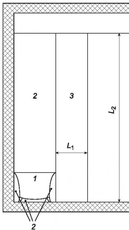
Рисунок 2 — Размеры зон: вид сбоку ванны
