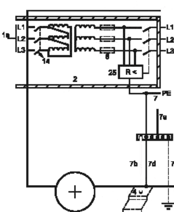
Рисунок 717.5 — Пример соединения с простым разделением и IT-системой с устройством контроля изоляции и отключением после первого замыкания на землю
