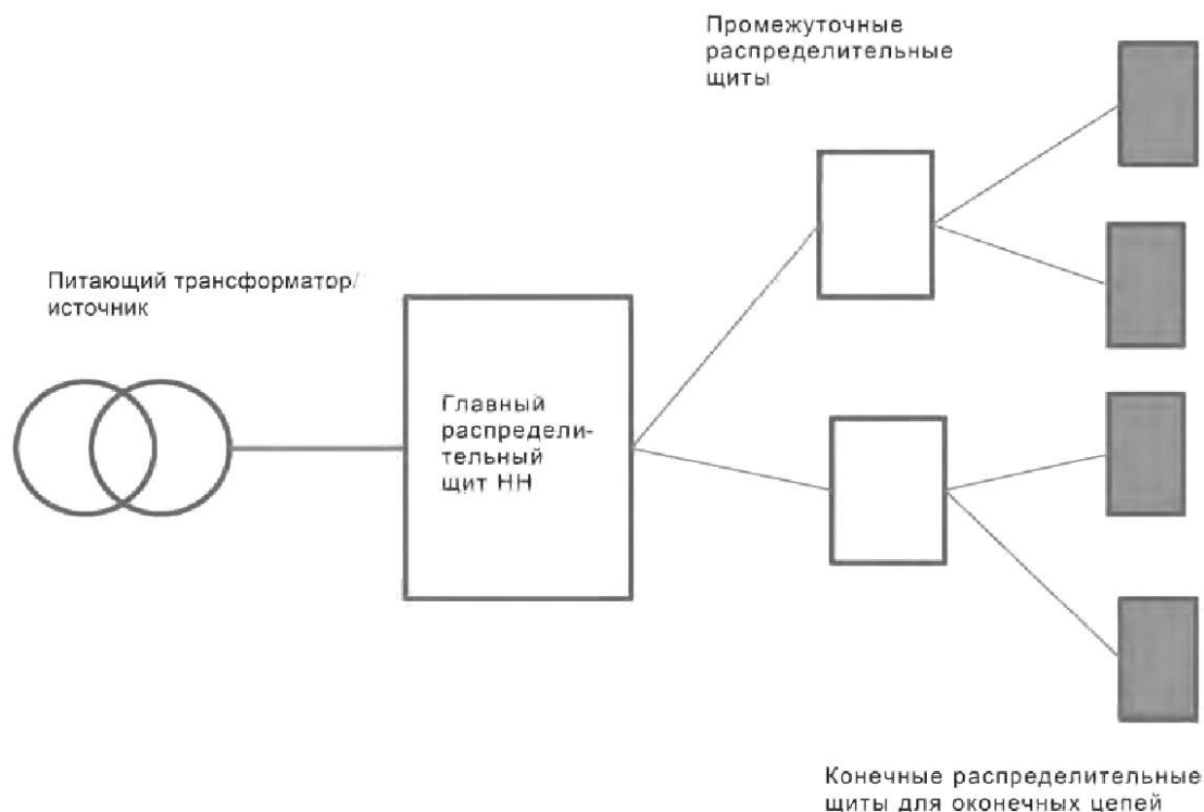
Рисунок 2 — Схема распределения мощности
