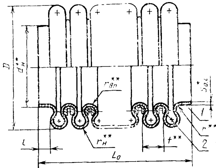
Рисунок 2 — Сильфон, тип 2
