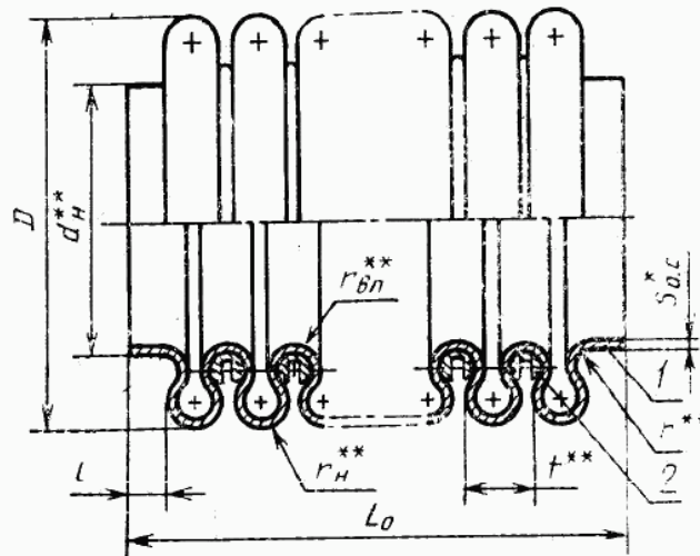
Рисунок 2 — Сильфон, тип 2
