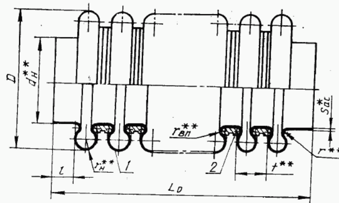
1—сильфон; 2—кольцо подкрепляющее
