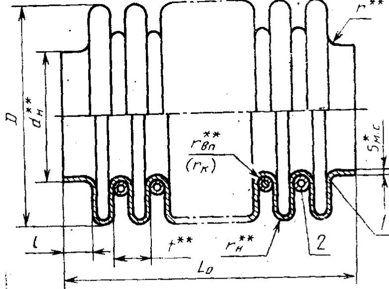
Рисунок 3 — Сильфон, тип 3
