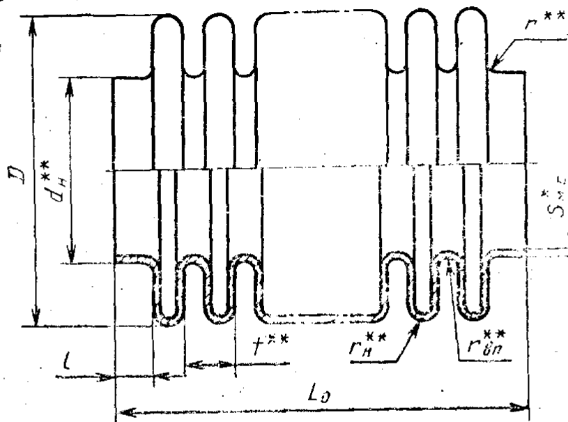
Рисунок 2 — Сильфон, тип 2
