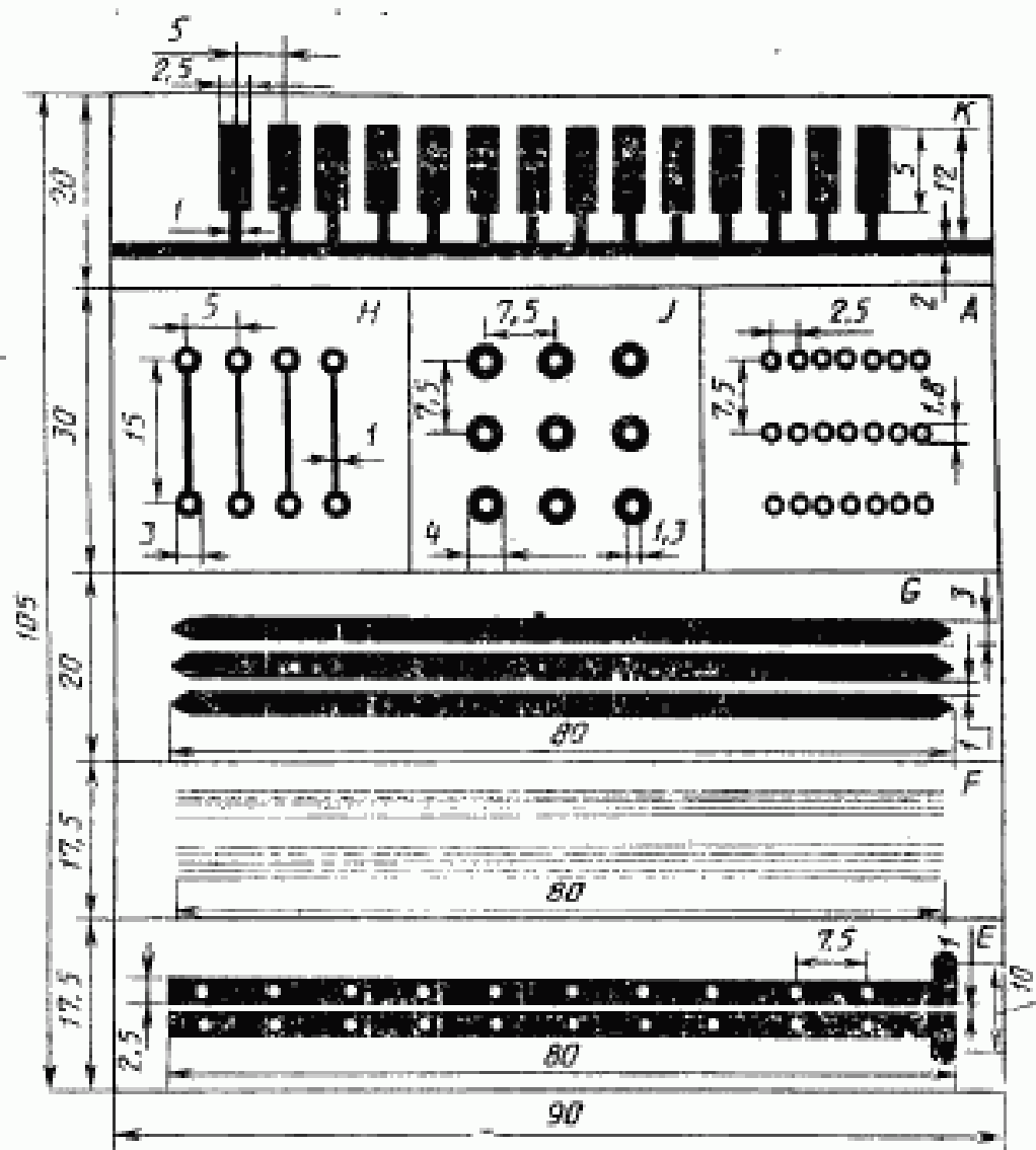
Рисунок 1 — Составной рисунок для испытаний
