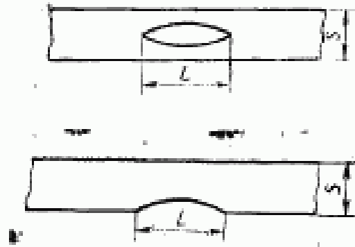
Рисунок 2 — Длина дефекта
