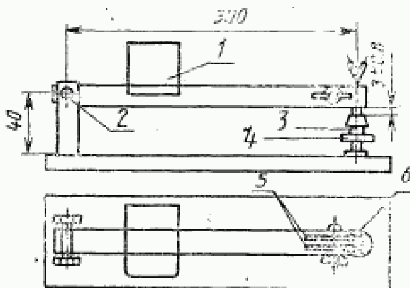
1—перемещающийся нос; 2—шарнирный валец; 3—патрон; 4—опора для патрона, чтобы рычаг находился в горизонтальном положении, когда усилие прилагают первый раз; 5—прорези в рычаге для более удобного вжима провода патрона; 6—отверстия для проводов
