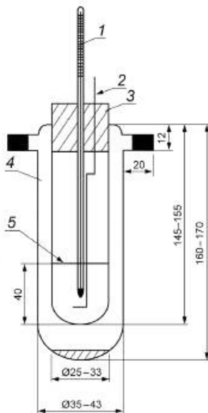
1 — термометр; 2 — мешалка; 3 — пробка; 4 — пробирка; 5 — кольцевая метка
