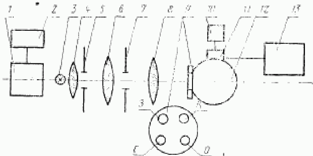
1 — стабилизатор напряжения; 2 — контрольный вольтметр (амперметр); 3 — лампа накаливания; 4 — конденсор; 5 — диафрагма; 6 — коллиматор; 7 — диафрагма; 8 — испытательный объект; 9 — турель с корректирующими светофильтрами; 10 — измерительный прибор; 11 — фотоприемник; 12 — фотометрический шар; 13 — высоковольтный стабилизатор напряжения
