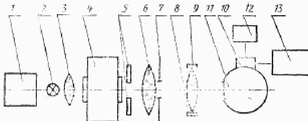
1 — стабилизатор напряжения; 2 — лампа накаливания; 3 — конденсор; 4 — монохроматор (или интерференционный светофильтр); 5 — светофильтр для устранения влияния вредного рассеянного света; 6 — коллиматор; 7 — диафрагма; 8 — объективодержатель; 9 — испытуемый объектив; 10 — фотоприемник; 11 — фотометрический шар; 12 — измерительный прибор; 13 — высоковольтный стабилизатор напряжения
