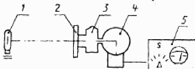
1 — нормированный источник света; 2 — объектив с/к; 3 — испытуемый фотоаппарат; 4 — светочувствительный фоток; 5 — контрольно-измерительный прибор
