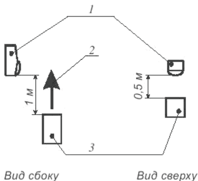
1 — ПОЗИИ; 2 — направление потока воздуха; 3 — тепловентилятор
