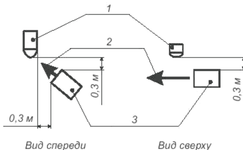
1 — ПОЗИИ; 2 — направление потока воздуха; 3 — тепловентилятор
