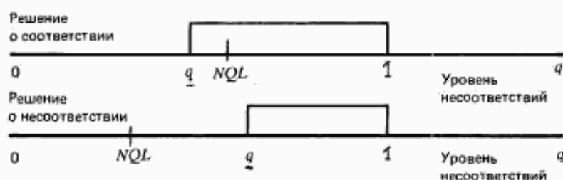
Рисунок 3 — Правила принятия решений при контроле потребителя по методу доверительных границ
