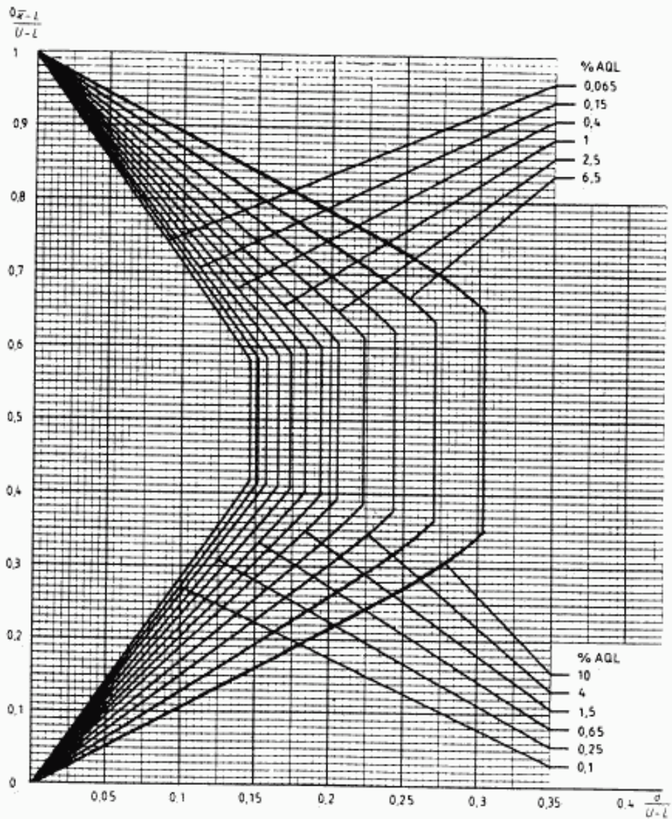
Диаграмма \sigma -P — Кривые приемки для предельных значений с общим уровнем качества: \sigma -метод для кода объема выборки P
