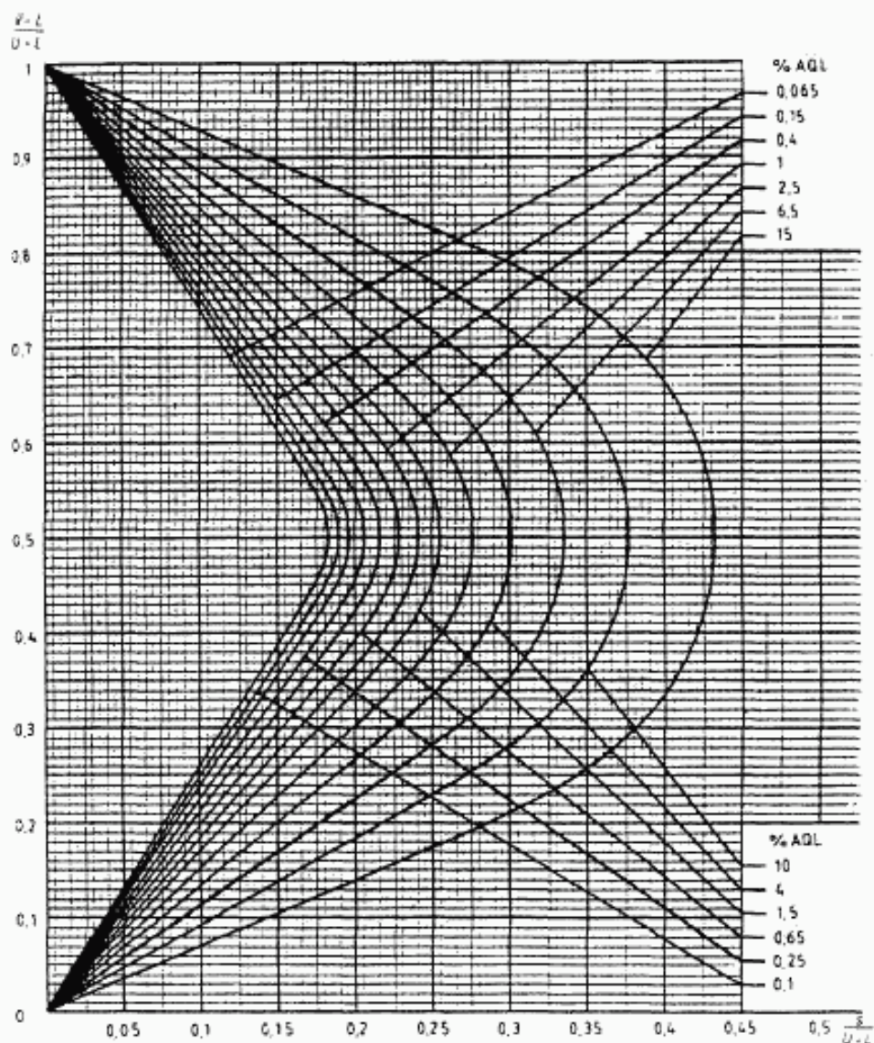
Диаграмма R-N — Кривые приемки для предельных значений с общим уровнем качества: R-метод для кода объема выборки N (объем выборки — 20)
