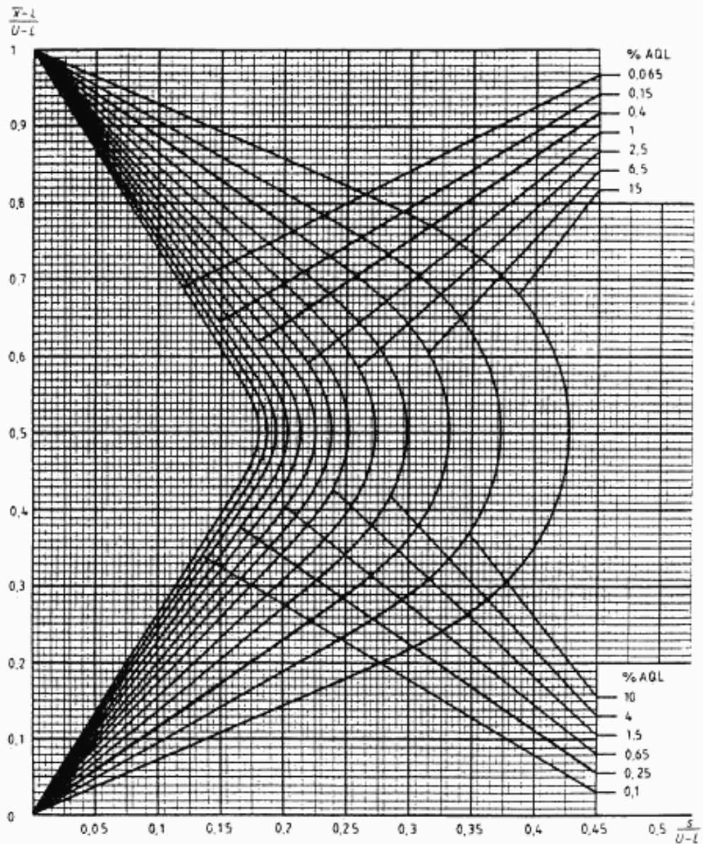
Диаграмма s-l — Кривые приемки для предельных значений с общим уровнем качества: s-метод для кода объема выборки I (объем выборки — 25)
