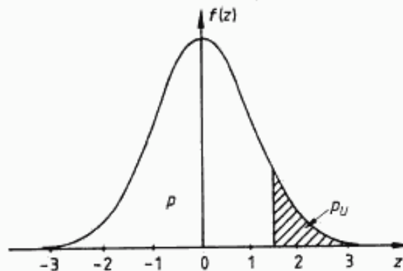
Рисунок 6 — Стандартное нормальное распределение
