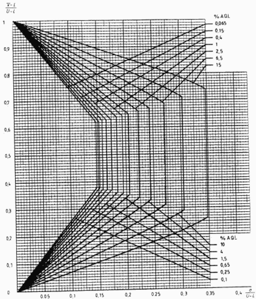
Диаграмма \sigma -I — Кривые приемки для предельных значений с общим уровнем качества: \sigma -метод для кода объема выборки I
