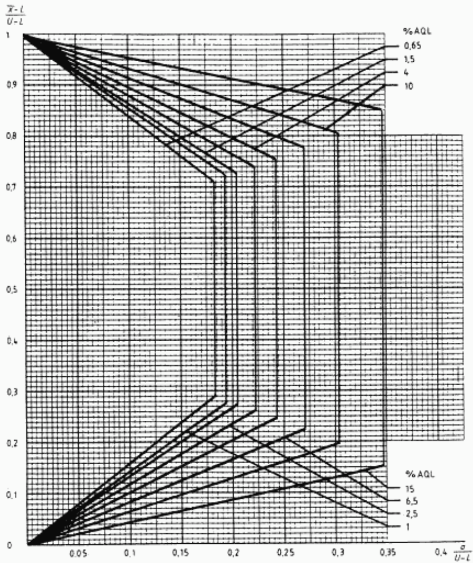
Диаграмма \sigma -D — Кривые приемки для предельных значений с общим уровнем качества: \sigma -метод для кода объема выборки D
