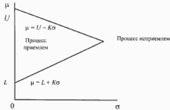
Рисунок 10 — Приемочная карта для двустороннего допуска ( \sigma и \mu известны)
