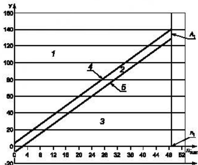
Рисунок 1 — Пример приемочной карты последовательного плана выборочного контроля для единственной границы допустимых значений
