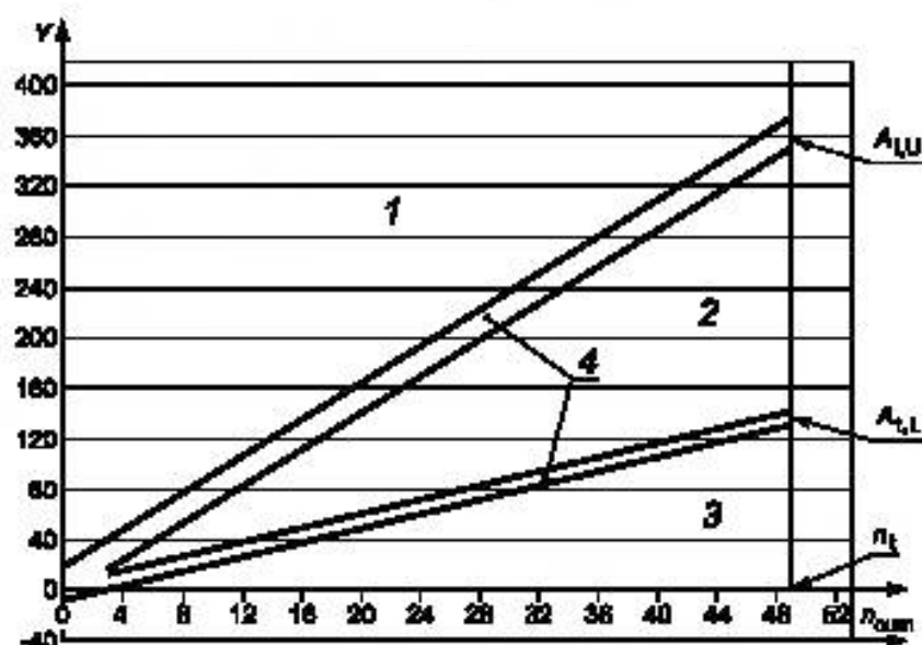
Рисунок 2 — Пример приемочной карты для последовательного плана объединенного контроля двух границ допустимых значений
