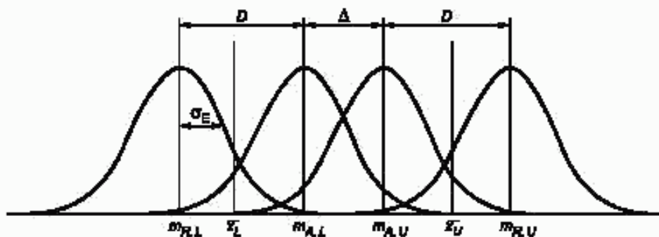
Рисунок С.3 — Соотношение между приемлемым уровнем качества и предельным уровнем качества и приемочными значениями \bar{x}_L , \bar{x}_U для двустороннего поля допуска
