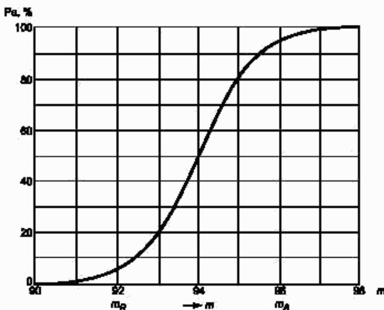
Рисунок D.4 — Оперативная характеристика для примера D.4
