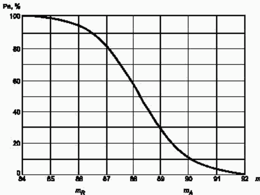
Рисунок D.2 — Оперативная характеристика для примера D.2
