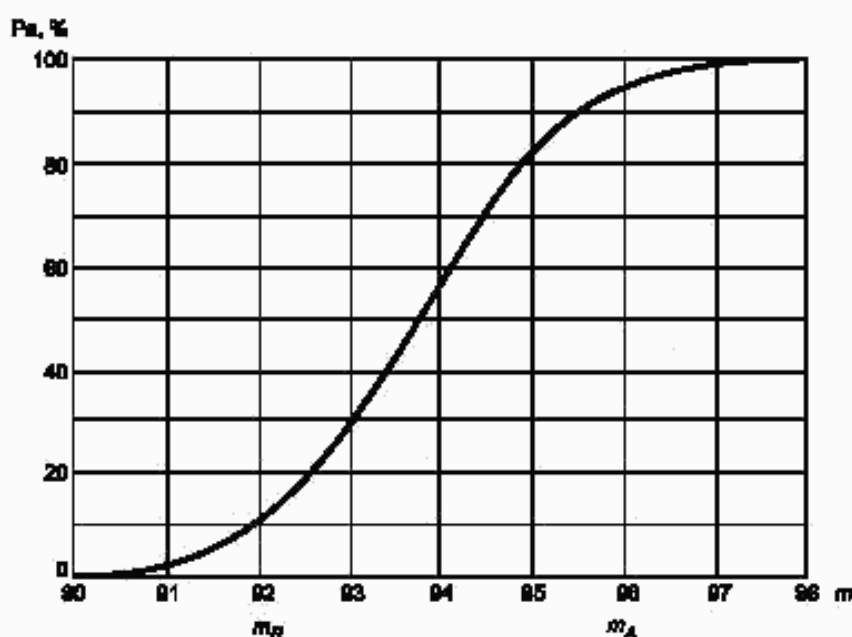
Рисунок D.1 — Оперативная характеристика для примера D.1
