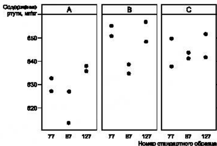
Рисунок А.2 — Результаты измерений содержания ртути в гипсе при анализе кандидата на стандартный образец
