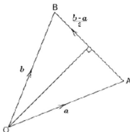
Рисунок 2 – Угол между двумя векторами
