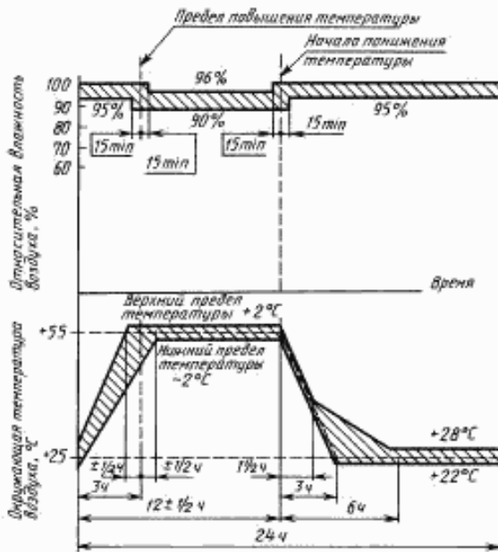
Рисунок 12 — Цикл испытания
