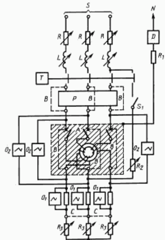
Рисунок 8 — Схема испытательной цепи для проверки правильности координации с аппаратом защиты от коротких замыканий и номинальной включающей и отключающей способности трехполюсного УЗО — D без встроенной защиты от коротких замыканий в трехфазной цепи
