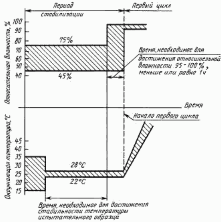
Рисунок 11 — Период стабилизации
