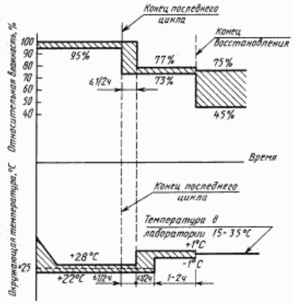
Рисунок 13 — Восстановление
