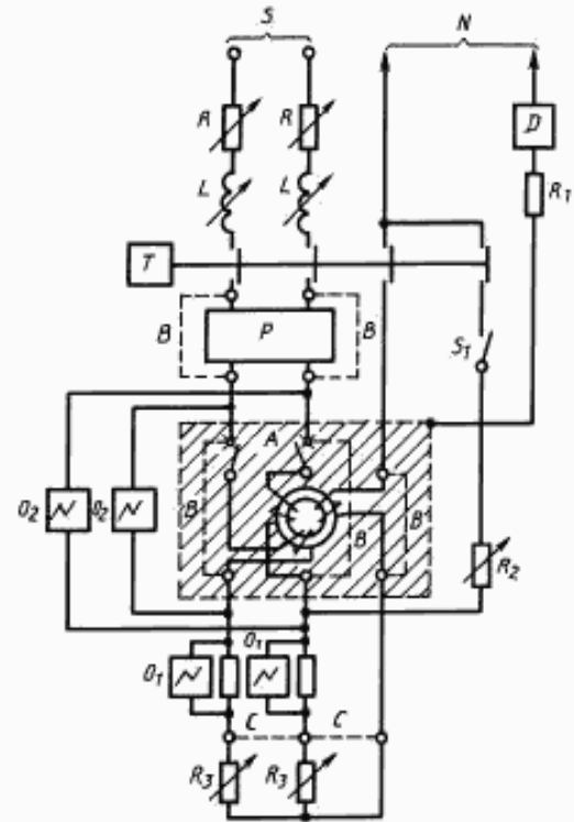
Рисунок 7 — Схема испытательной цепи для проверки правильности координации с аппаратом защиты от коротких замыканий и номинальной включающей и отключающей способности двухполюсного УЗО — D с тремя путями прохождения тока без встроенной защиты от коротких замыканий в однофазной цепи со средней нейтралью
