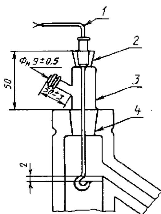
1 — термопара; 2 — конус 14/20; 3 — переходная муфта; 4 — конус 19/38
