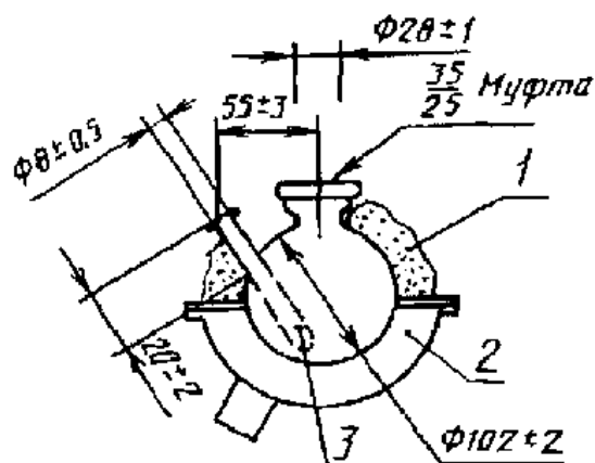
1 — теплоизоляционный материал; 2 — нагреватель; 3 — карман термопары
