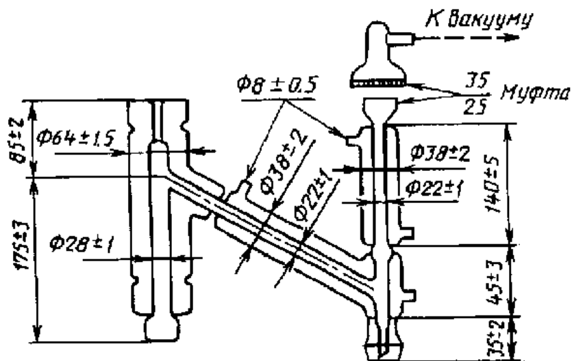
Рисунок 3 — Колонка с вакуумной рубашкой
