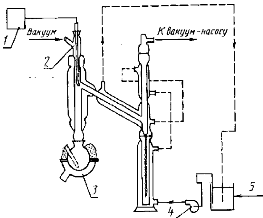
1 — потенциометр; 2 — переходник для термопары; 3 — нагреватель; 4 — насос; 5 — термостат
