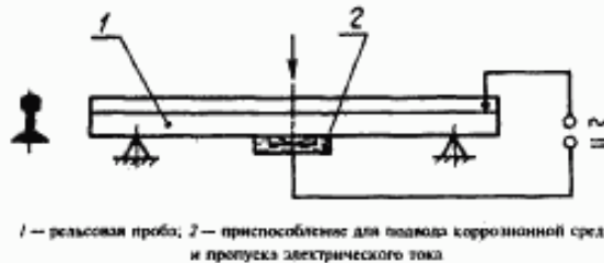
Рисунок 2 — Схема испытания рельсовых проб на коррозионную усталость
