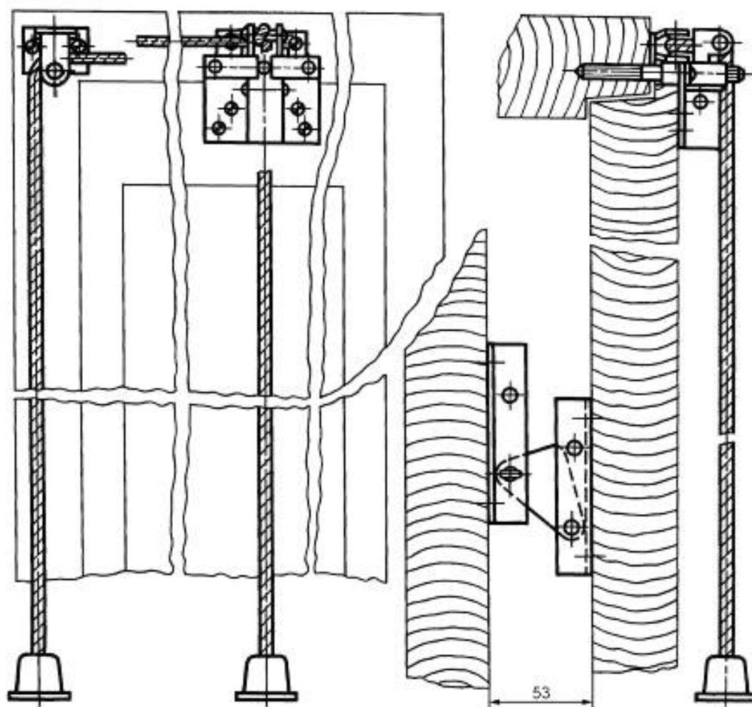
Рисунок В.2 — Фрамужный прибор типа ПФ-2
