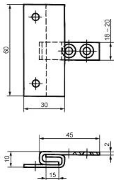
Рисунок Б.2 — Соединитель для фрамуг с тройным остеклением
