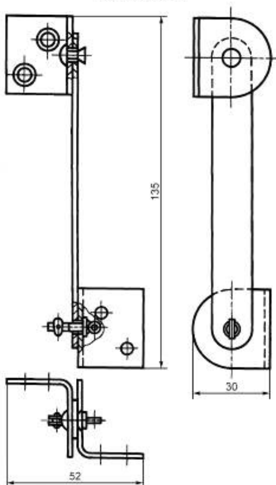
Рисунок Б.1, лист 2
