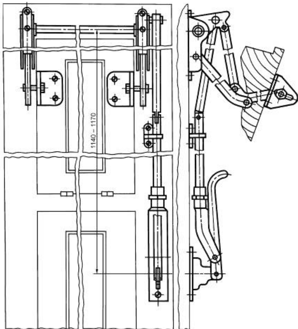
Рисунок В.1 — Фрамужный прибор типа ПФ-1
