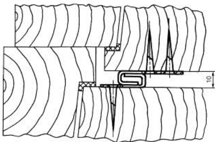
Рисунок В.3 — Фрамужный соединитель типа СФ-2
