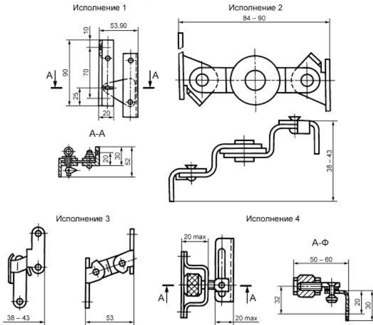
Рисунок Б.1 — Соединители для фрамуг с отдельными и раздельно-спаренными переплетами
