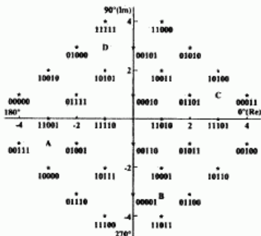
Рисунок 2 — Сигнальное созвездие КАМ-32 для скорости 9600 бит/с
