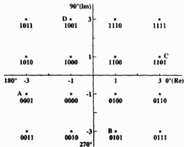
Рисунок 1 — Сигнальное созвездие КАМ-16 для скорости 9600 бит/с
