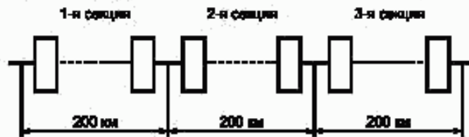
Рисунок Б.1 – ГЭЦТ длиной 600 км
