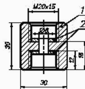
1 — переходник; 2 — прокладка
