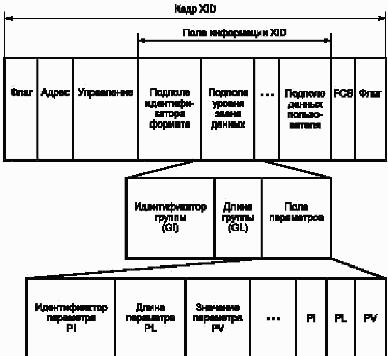
Рисунок 3 — Общий формат поля информации XID
