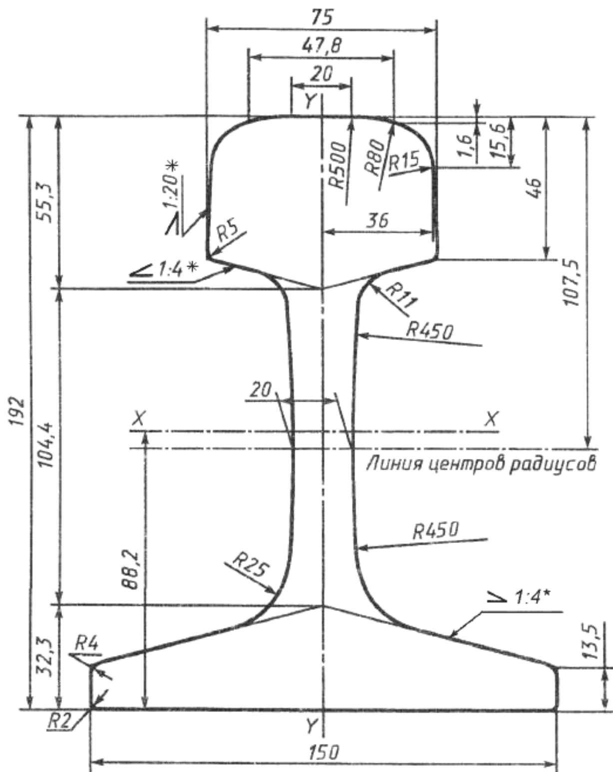
Рисунок А.5 – Рельс типа РП75
