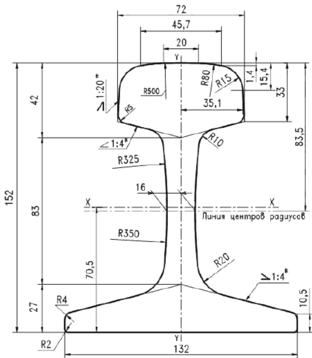
Рисунок А.1 – Рельс типа РП50
