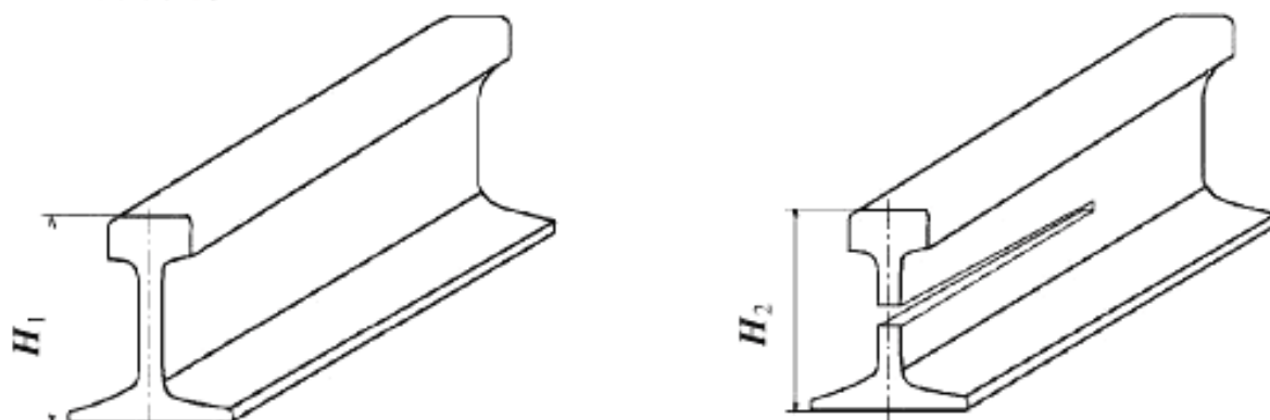
Рисунок 4 – Схема определения остаточных напряжений в шейке рельсов
