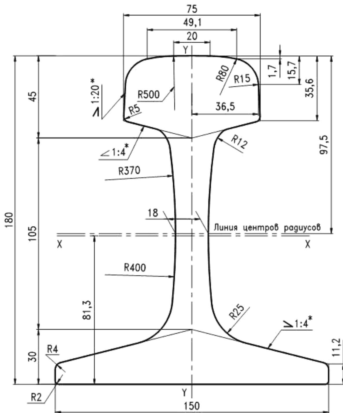
Рисунок А.3 – Рельс типа РП65
