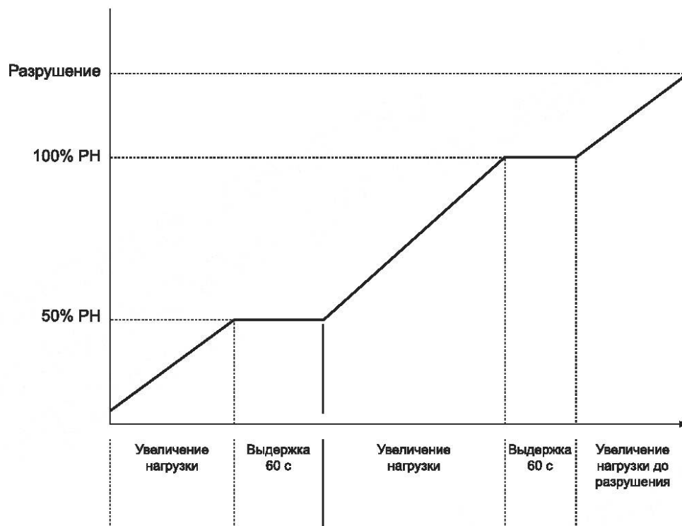
Рисунок 3 — Механическое испытание при разрушающей нагрузке (PH)
