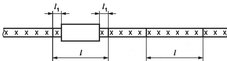
Рисунок 12 — Схема измерения сопротивления электрического контакта
