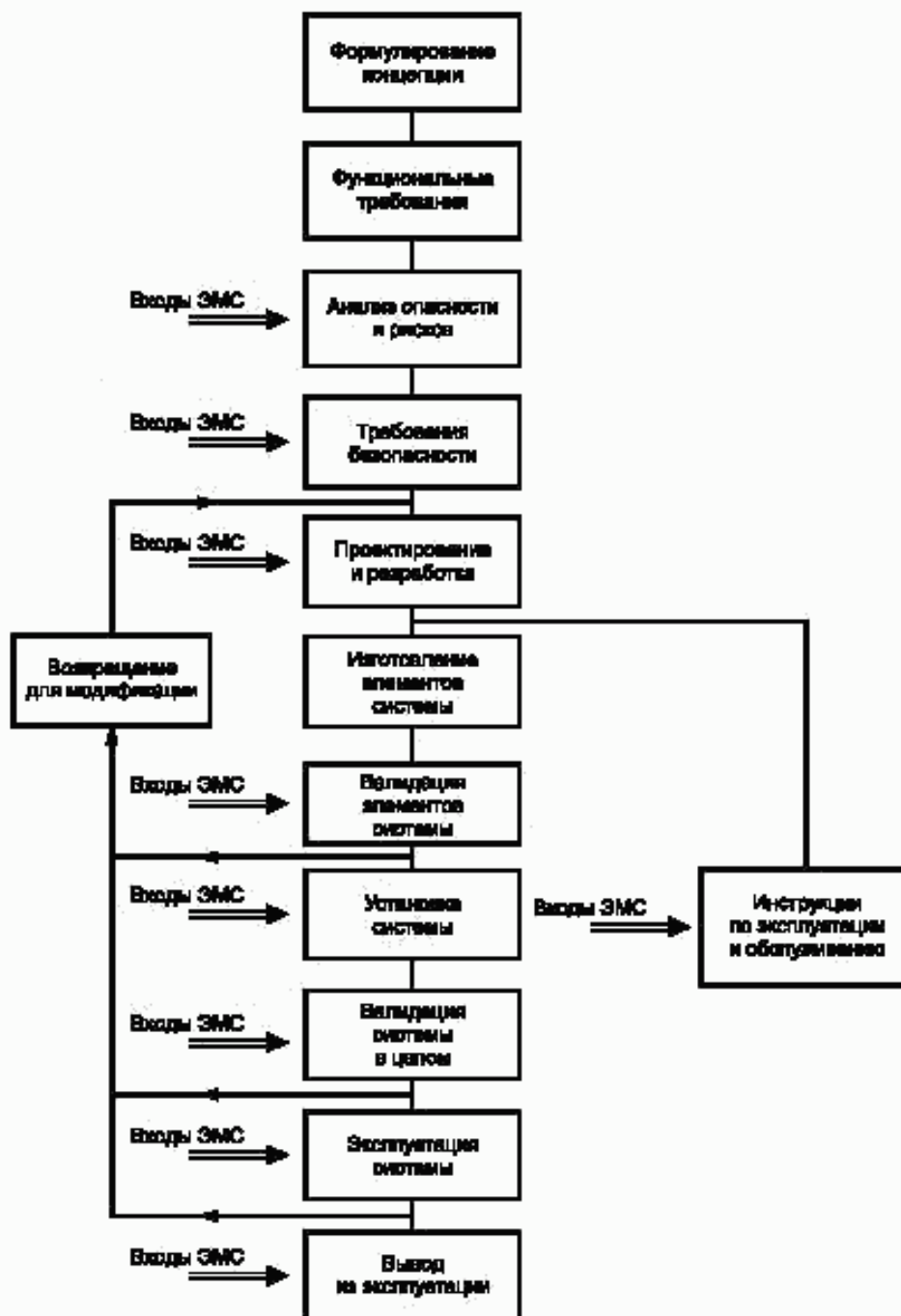
Рисунок 2 — Схема обеспечения функциональной безопасности применительно к стадиям жизненного цикла системы
