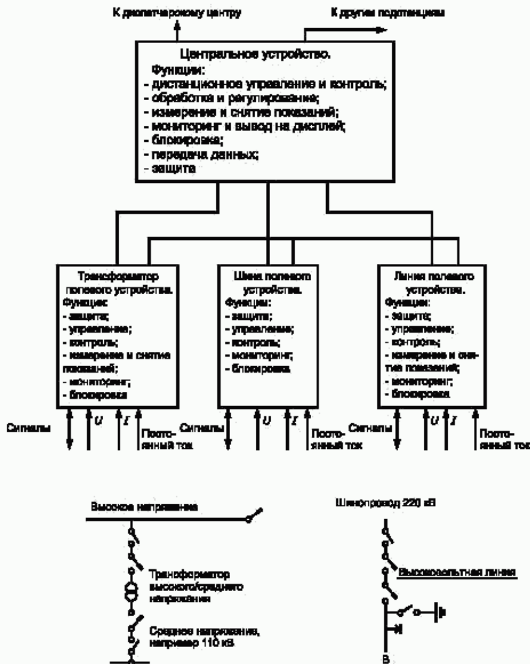
Рисунок Б.5 — Общая структура системы контроля и управления высоковольтной подстанции
