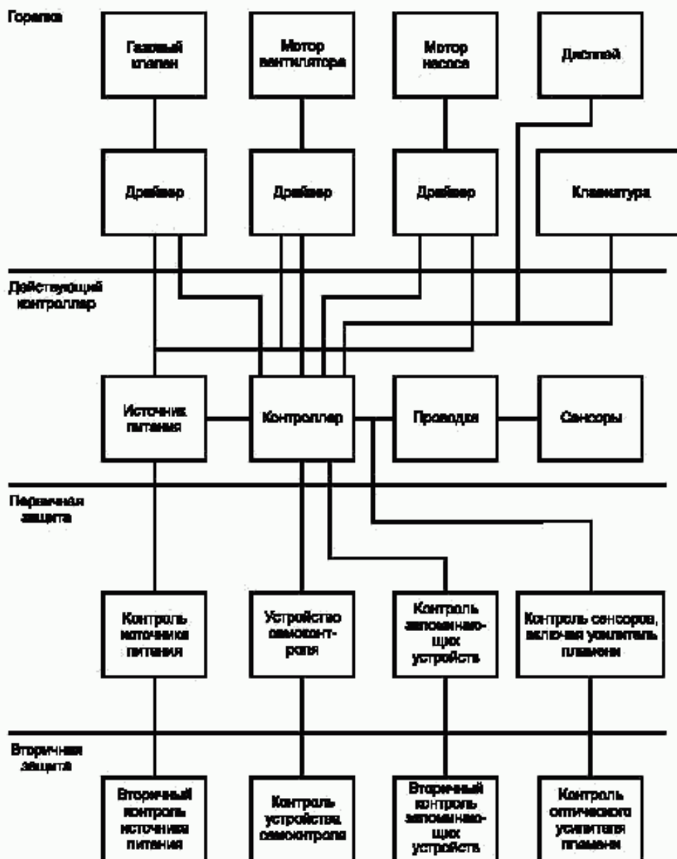
Рисунок Б.3 — Контроллер газовой горелки: блок-схема
