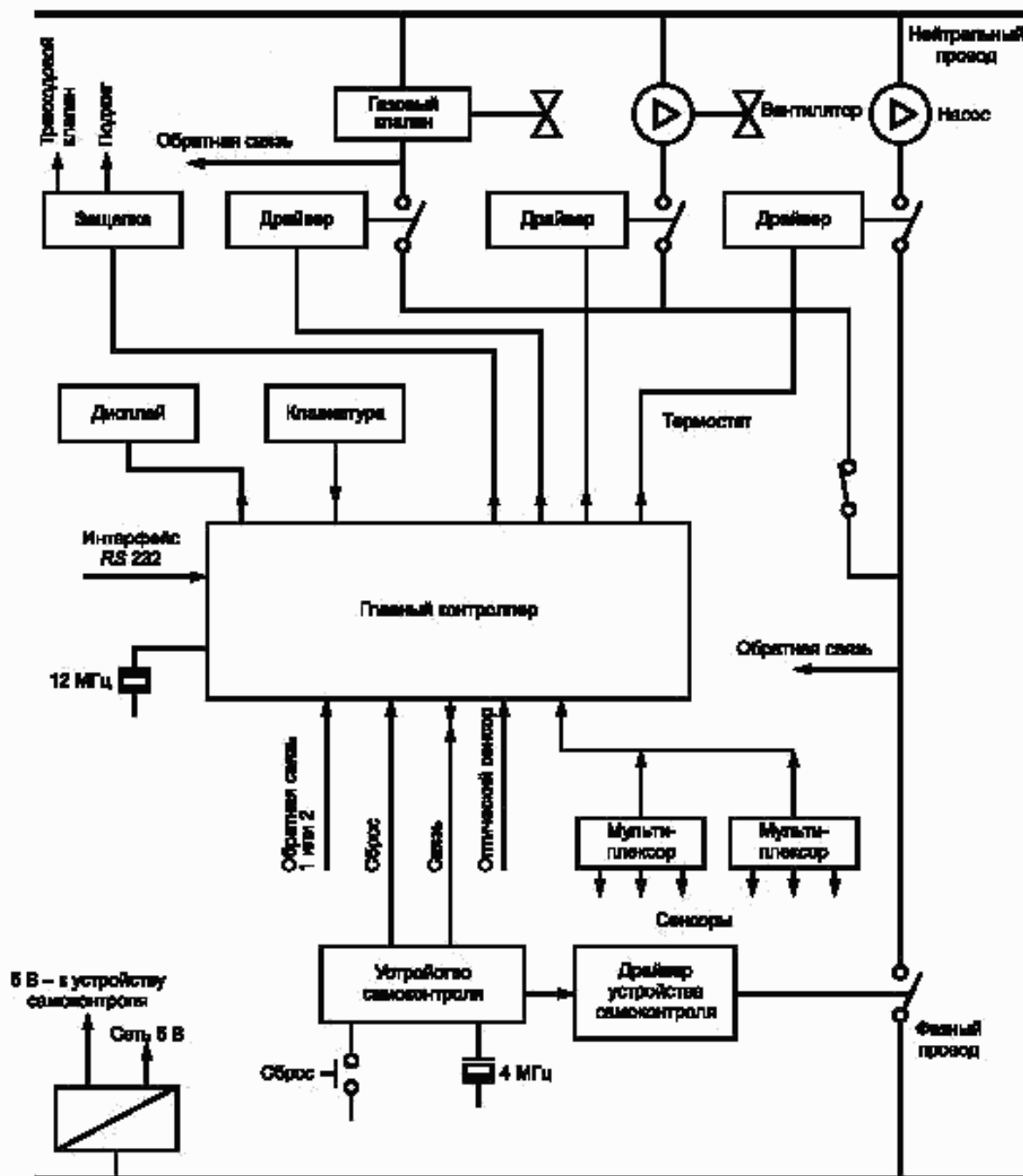
Рисунок Б.2 — Контроллер газовой горелки: структура
