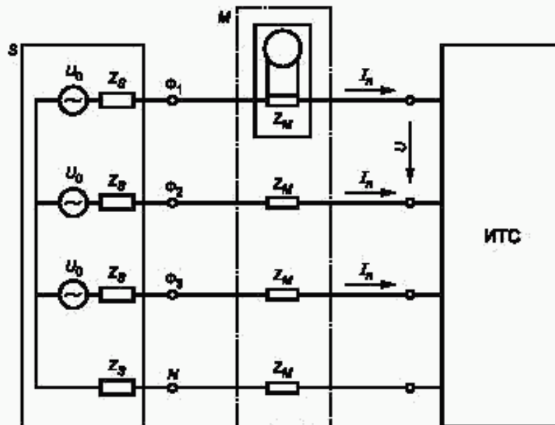
Рисунок А.1 — Схема измерений для однофазных ТС
