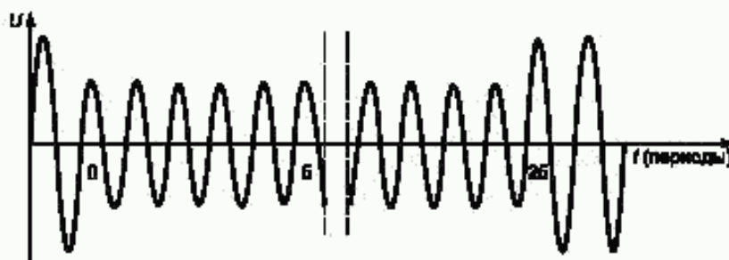
Рисунок 1 — Провал напряжения 70 % U_T
