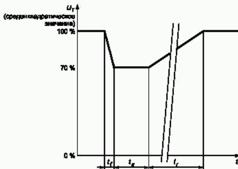
Рисунок 1 — Провал напряжения 70 % U_T
