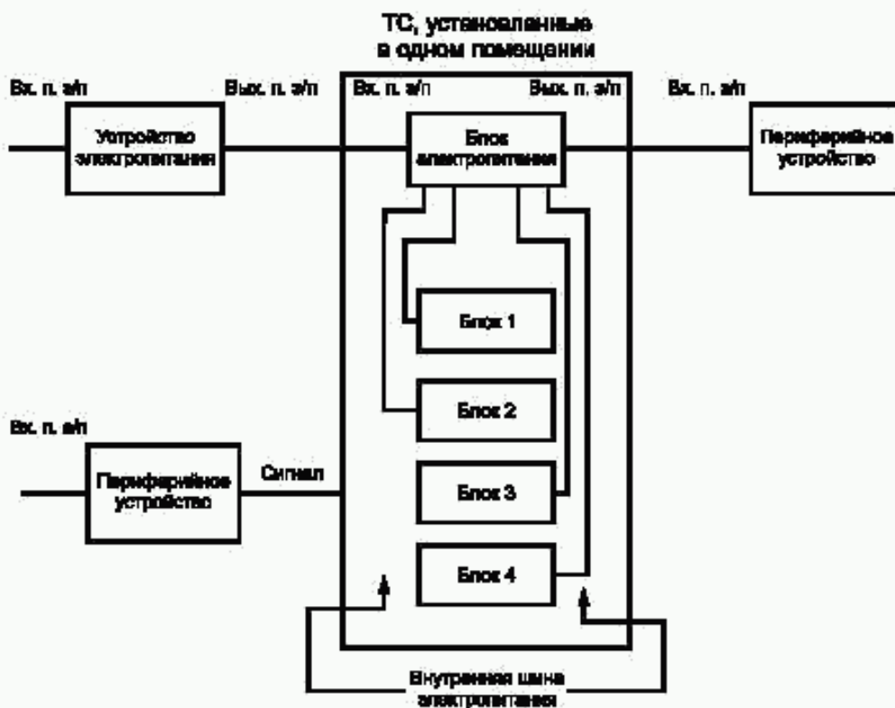
Рисунок 2 — Примеры портов электропитания
