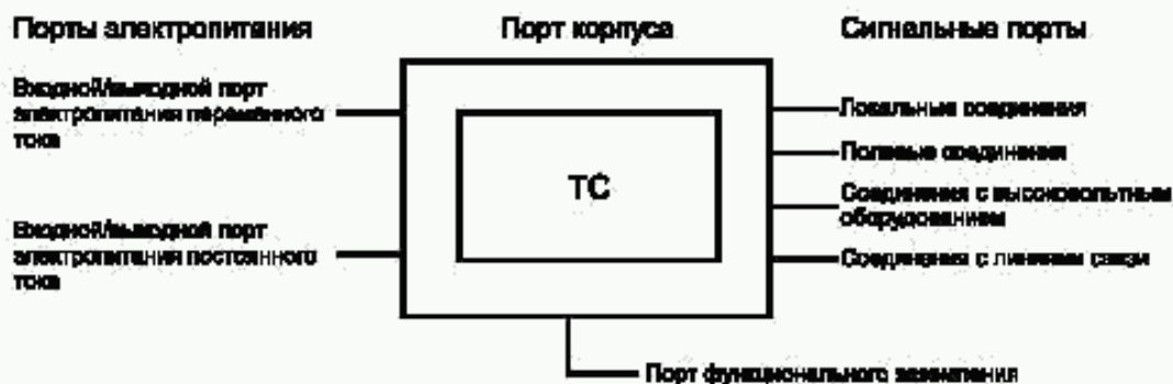
Рисунок 1 — Порты ТС
