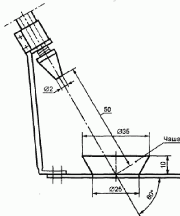
Рисунок 4 — Разбрызгиватель
