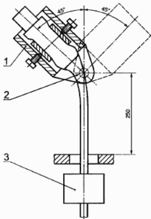
1 — устройство крепления образца; 2 — ось колебаний; 3 — груз
