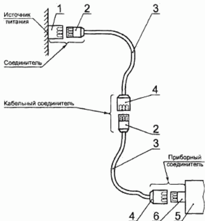
Рисунок 1 — Схема применения соединителя
