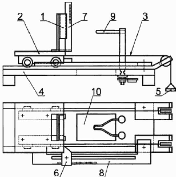
Рисунок 9 — Устройство для испытания на изгиб
