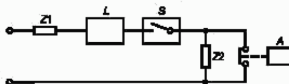
Z1 — сопротивление для регулировки ожидаемого тока короткого замыкания (безиндуктивное); Z2 — сопротивление для регулировки нагрузки (безиндуктивное); L — ограничивающее устройство для величины I^2t ; S — испытуемый образец; A — вспомогательный выключатель для создания короткого замыкания
