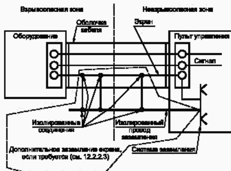
Рисунок 2 — Заземление проводящих экранов
