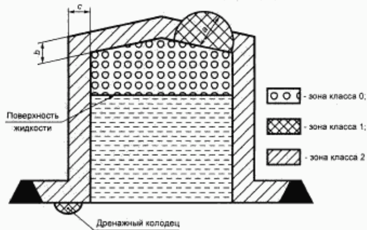
Пример № 8 Резервуар для хранения горючей жидкости, установленный снаружи, с неподвижной крышей и без внутренней плавающей крышки
