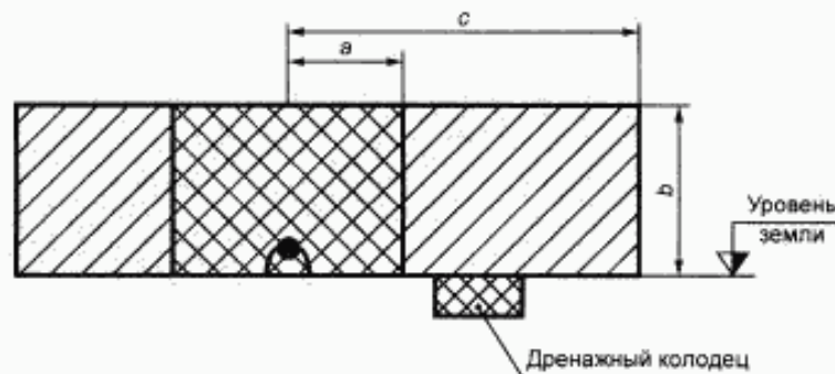
Пример № 2 Насос для перекачки горячей жидкости, установленный снаружи на уровне земли
