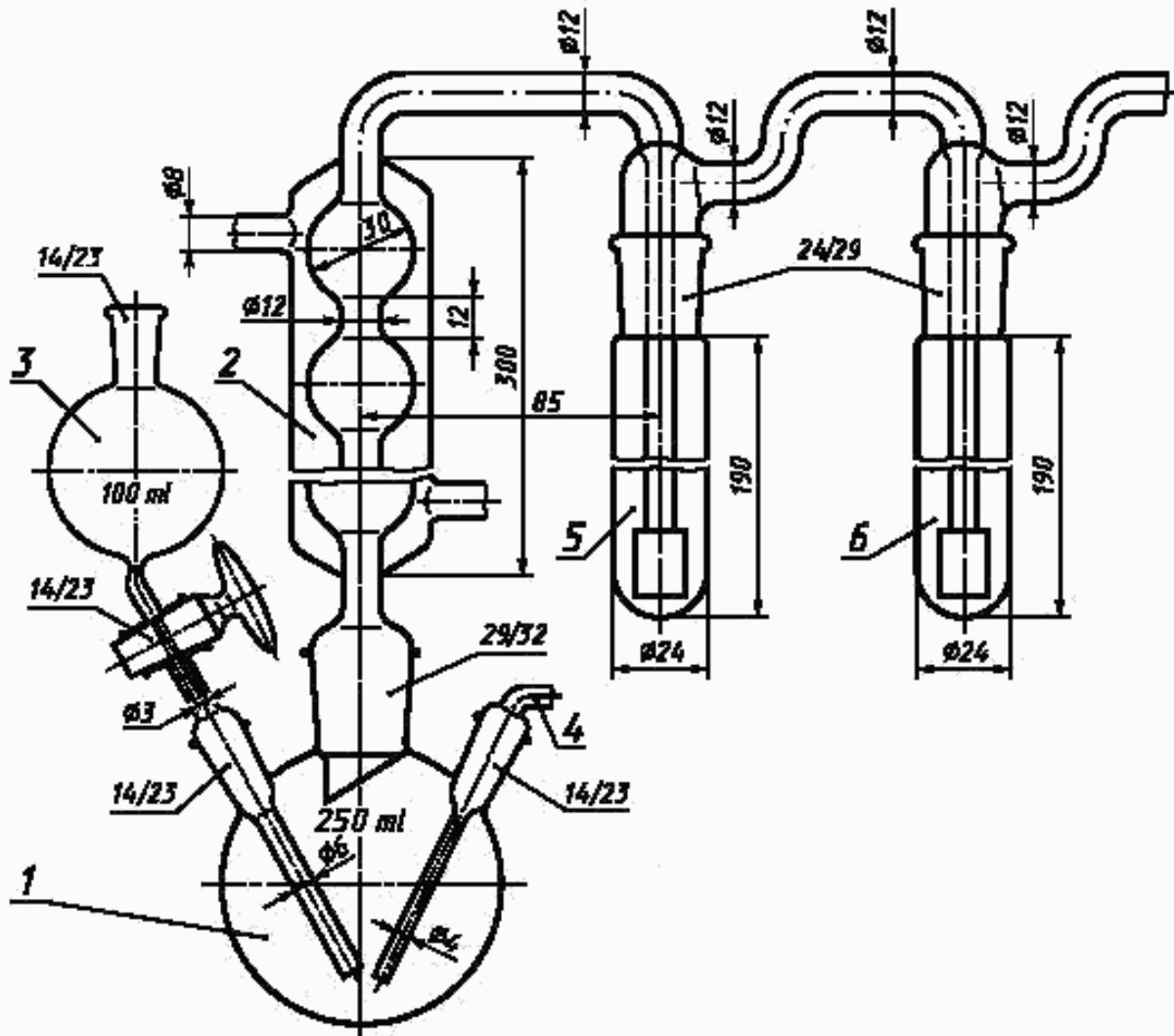
1 — дистилляционная колба; 2 — обратный холодильник; 3 — капельная воронка; 4 — подводная трубка; 5 и 6 — газопоглощающие устройства
