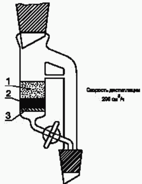
1 — табак + Флоризил®; 2 — флоризил®; 3 — пористая фильтрующая пластина № 1 размером пор 100—120 мкм
