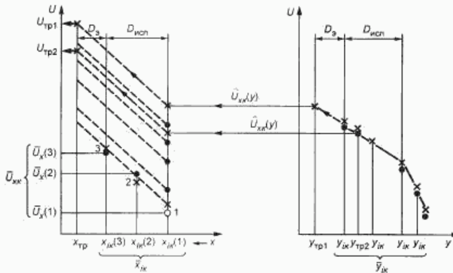
Рисунок А.4 — Схема эксперимента по варианту 4
