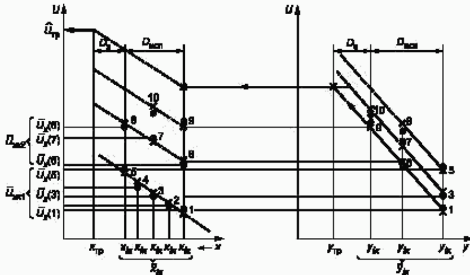
Рисунок А.3 — Схема эксперимента по варианту 3
