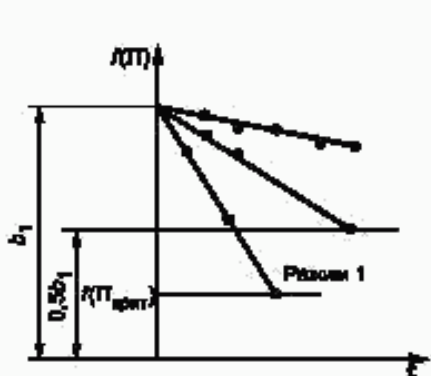
Рисунок Б.1 — Скорость изменения значения параметра в процессе испытания, неизменная
