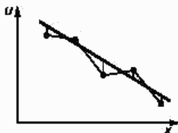
Рисунок Д.2 — Пример приемлемости гипотезы линейности при F_{табл} < F
