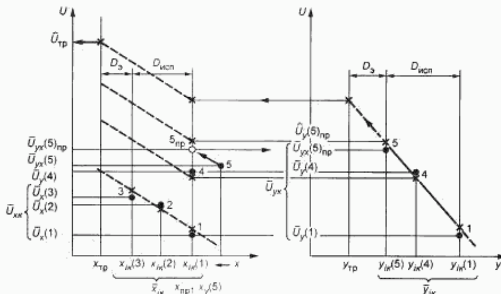
Рисунок А.2 — Схема эксперимента по варианту 2
