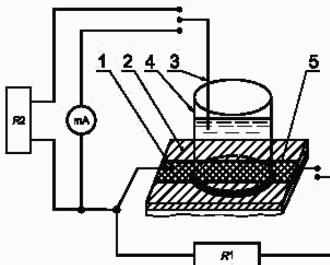
1 — тонкий слой железа; 2 — лакокрасочное покрытие; 3 — платиновый электрод; 4 — стаканчик с подкисленной водой; 5 — пластилин; R1 — мост постоянного тока МО-62; R2 — термометр МОИ-4; mA — миллиамперметр М-95
