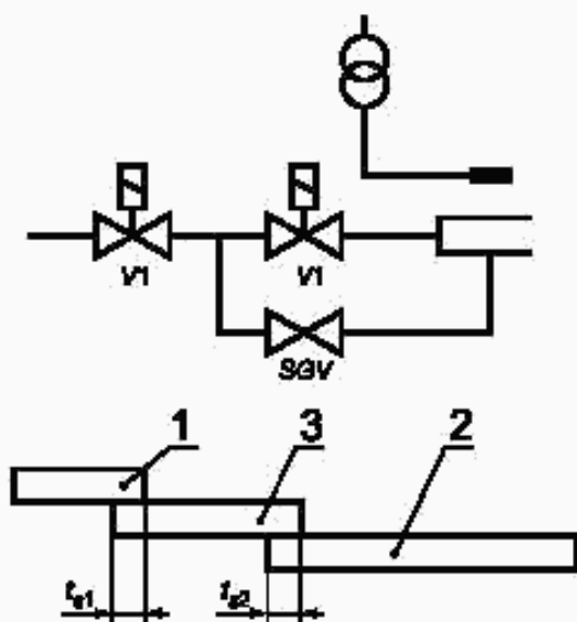
VI — основной предохранительный газовый отсечной клапан; SGV — предохранительный отсечной клапан подачи пускового газа; t_{s1} — первое время безопасности; t_{s2} — второе время безопасности; 1 — зажигание; 2 — основная горелка; 3 — пусковой газ
