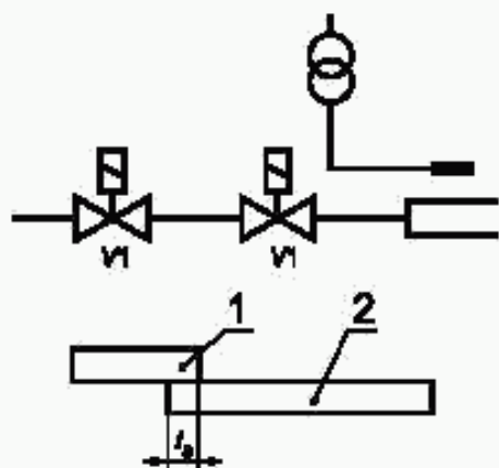
VI — основной предохранительный отсечной газовый клапан; t_s — время безопасности; 1 — зажигание; 2 — основная горелка
