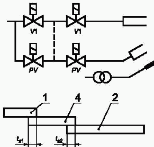
VI — основной предохранительный газовый отсечной клапан; PV — предохранительный отсечной клапан запальной горелки; t_{s1} — первое время безопасности; t_{s2} — второе время безопасности; 1 — зажигание; 2 — основная горелка; 4 — пилот
