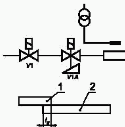
VI — основной предохранительный отсечной газовый клапан; VIА — основной предохранительный отсечной газовый клапан медленного открытия; t_s — время безопасности; 1 — зажигание; 2 — основная горелка
