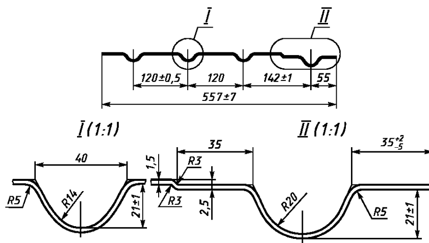
Рисунок 4 — Профиль 557-21-1,5, ГЛ4-238
