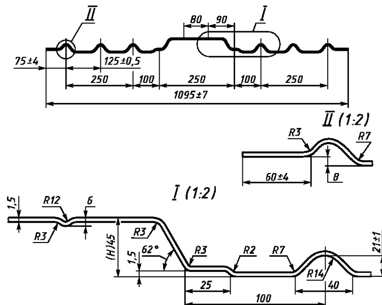
Рисунок 2 — Профиль 1095·45·21·1,5, ГЛ4-220А
