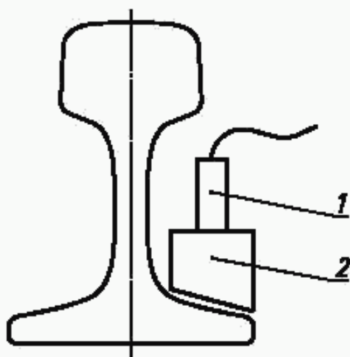
1 — датчик; 2 — переходник
